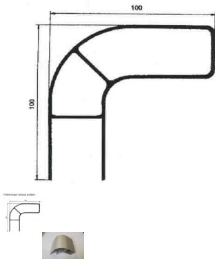
Fietsenvanger verticale profielen
